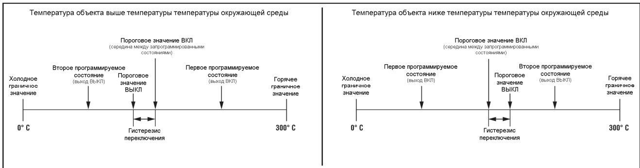
Рис. 3 Статический 2-х точечный режим программирования
