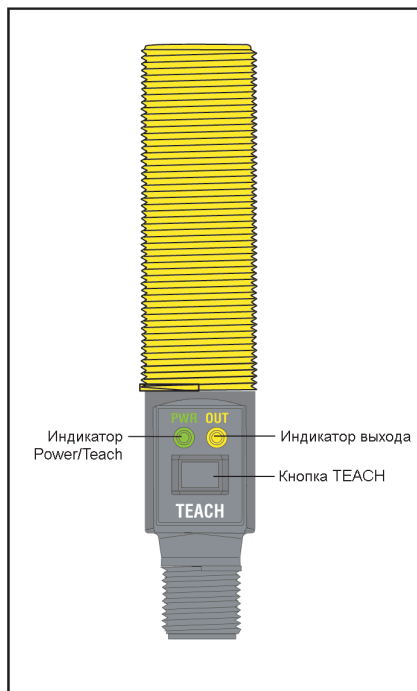
Рис. 1. Вид датчика
